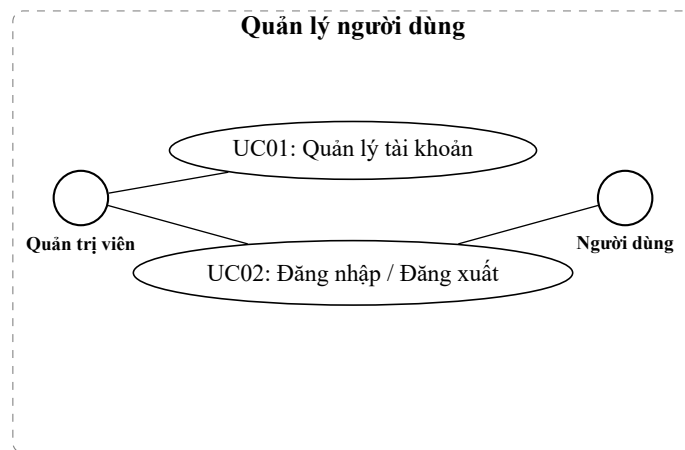
Hình 1: Sơ đồ use case phân rã – Quản lý người dùng
